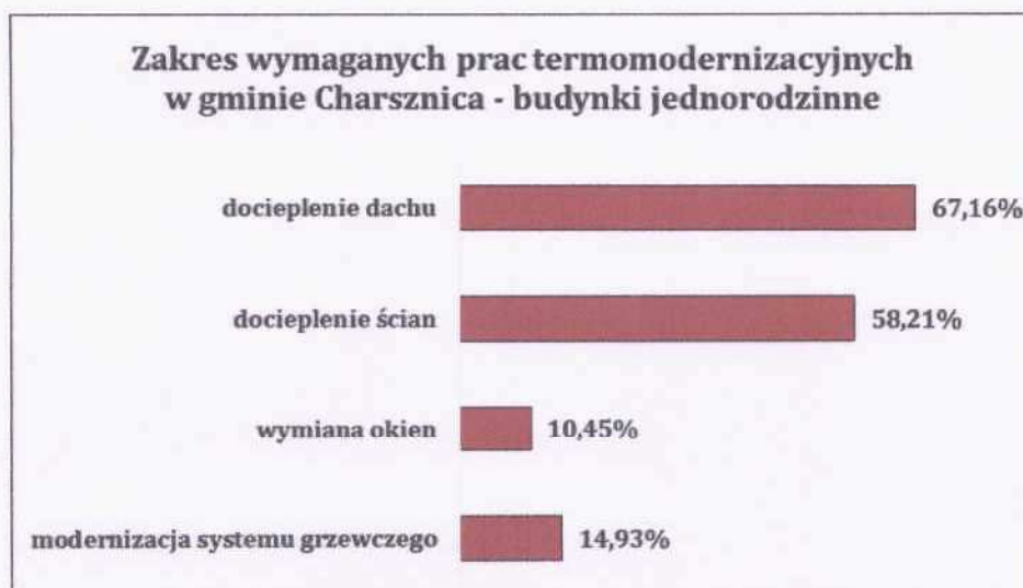
Wykres 7 Zakres prac termomodernizacyjnych potrzebnych w budynkach jednorodzinnych [Ankietyzacja]
